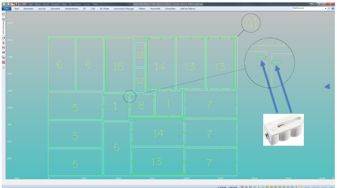
Verschachtelte Bauteile von Schränken mit Cabineo Verbinder.
